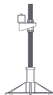
Base y Long Stud Leg Assembly Ajuste de altura: 335 - 660mm
