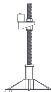
Piastre Long Stud Altezza di regolazione: 335 - 660 mm
