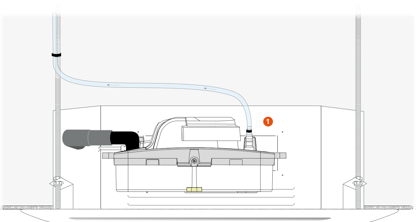
1 Max Hi-Flow geschroefd op cassette-unit
