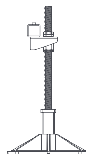
Удлиненная нога в сборе Высота 335-660 мм
