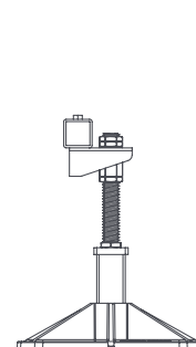
Стандартная сборка Высота 335-440 мм
